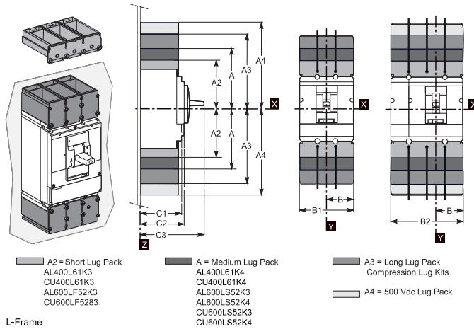
L-Frame
